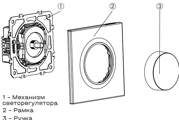
Рис. 2. Схема сборки
