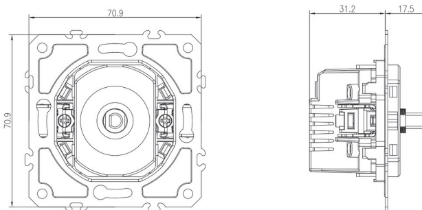
Рис. 1. Габаритные размеры
