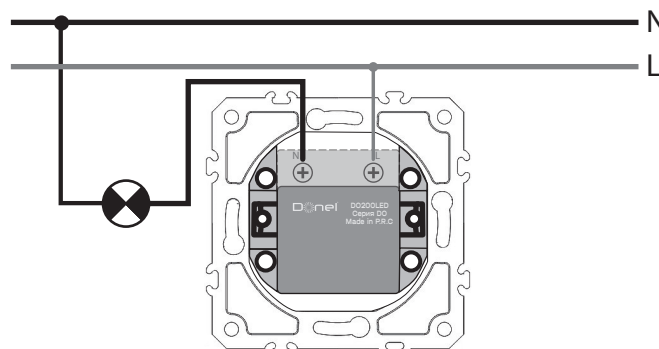
Рис. 3. Схема подключения светорегулятора
