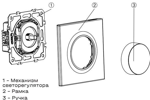
Рис. 2. Схема сборки
