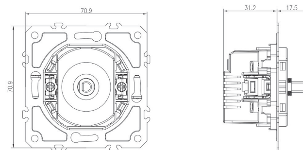
Рис. 1. Габаритные размеры
