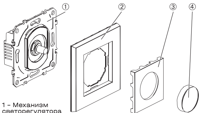
Рис. 2. Схема сборки
