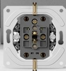
Механизм двойной розетки с заземлением
