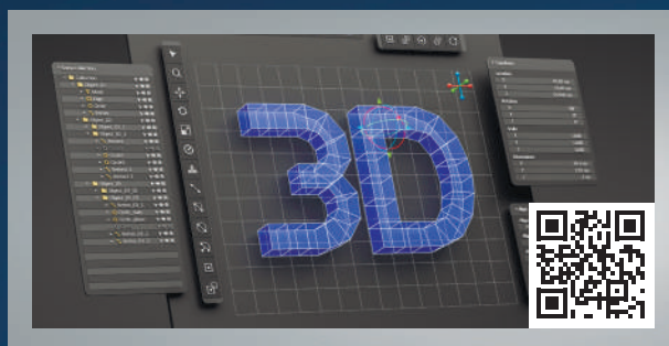
3D МОДЕЛИ
